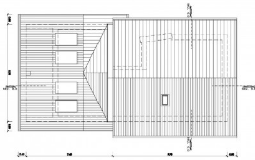
PIANTA COPERTURA
