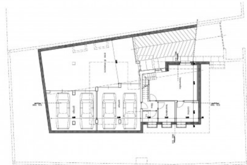
PIANTA PIANO INTERRATO
