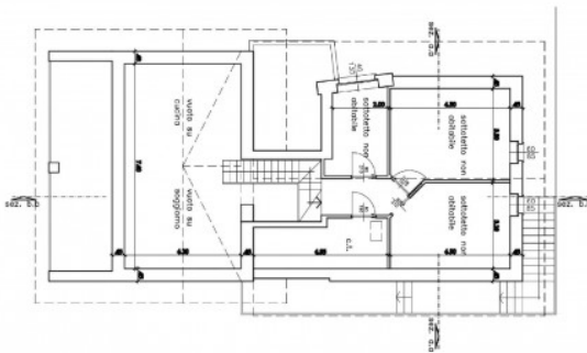
PIANTA PIANO SOTTOTETTO
