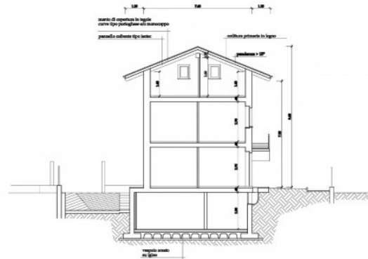
SEZIONE A-A
