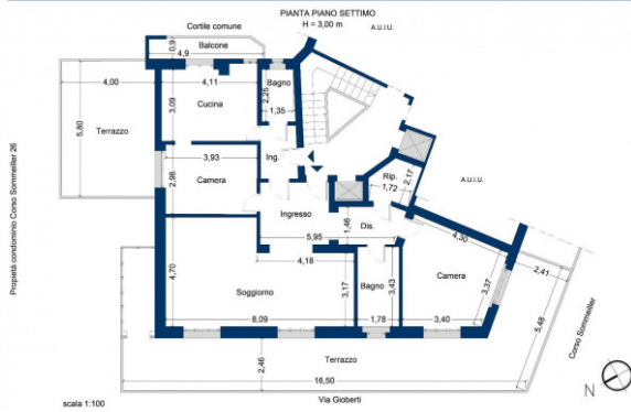
Planimetria unità immobiliare Corso Sommeiller 26 - Torino
